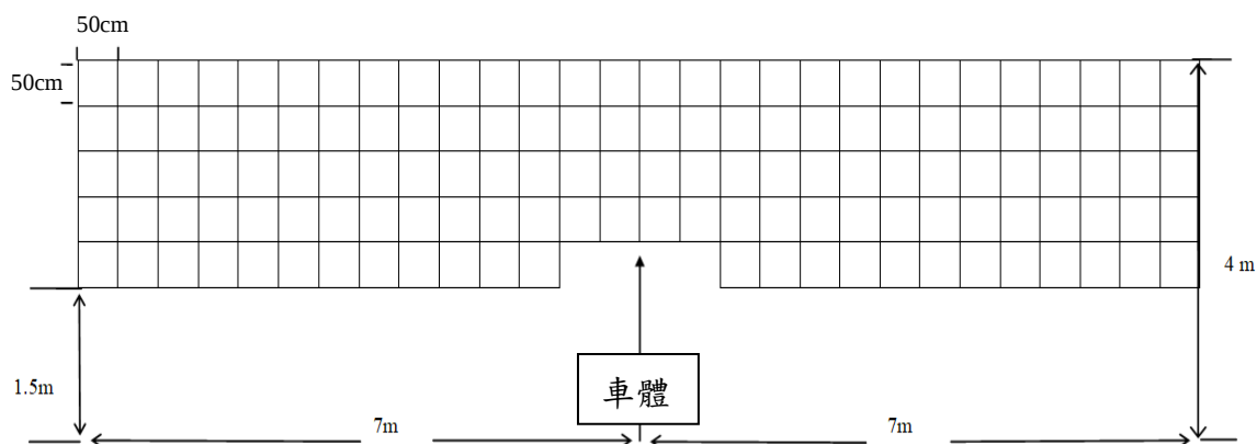
附圖三、實際撒佈性能測定所用撒佈網規格
