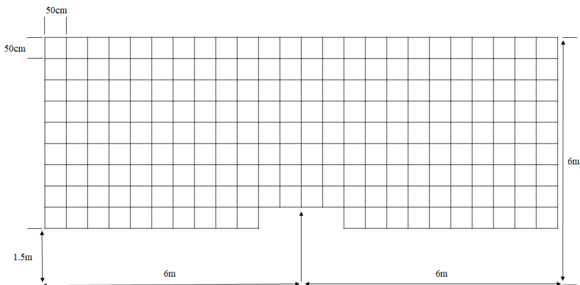
附圖二、撒佈性能測定所用撒佈網規格
