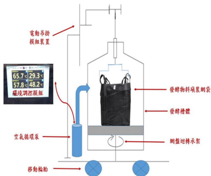
固態發酵裝置組裝示意圖
