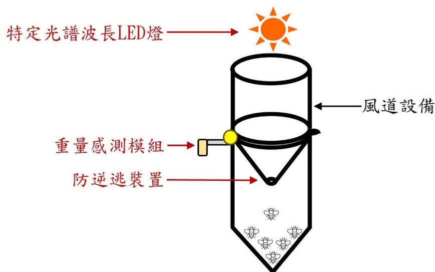
捕蟲裝置示意圖
