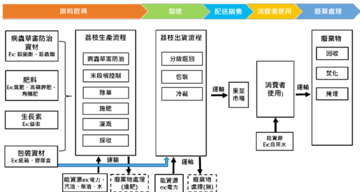
玉荷包荔枝碳盤查之生命週期流程圖。
