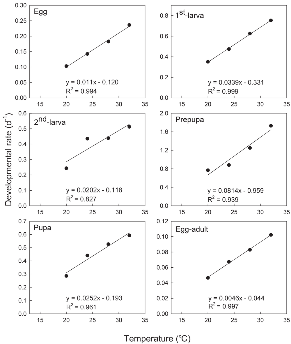
圖 1. 溫度與檬果上小黃薊馬發育速率之直線關係。
